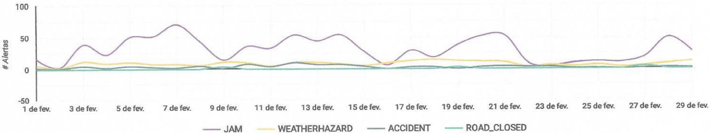
Número de Alertas por subtipo O gráfico a seguir ilustra o número de alertas por dia, discriminados por subtipo de alerta. Todos os subtipos podem ser encontrados no Dicionário de dados Página Inicial .
